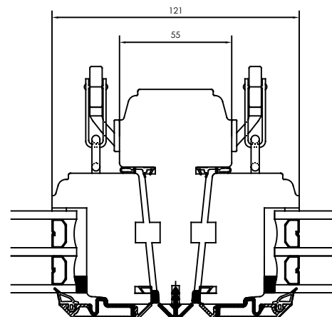
Horizontalsnitt 2-luft Horizontal section 2-lights
