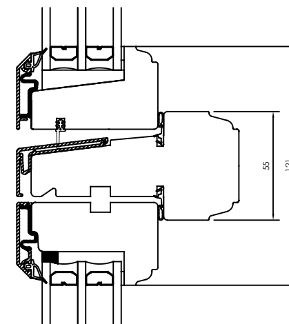
Vertikalsnitt 2-luft Vertical section 2-lights
